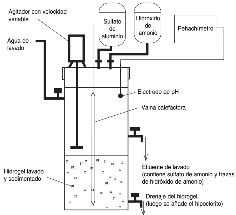
FIGURA 1. Representación esquemática de la preparación del hidrogel de hidróxido de aluminio a escala piloto
