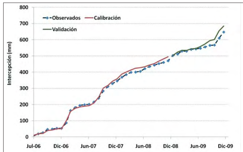
Figura 12. Ajuste del modelo de redistribución.
