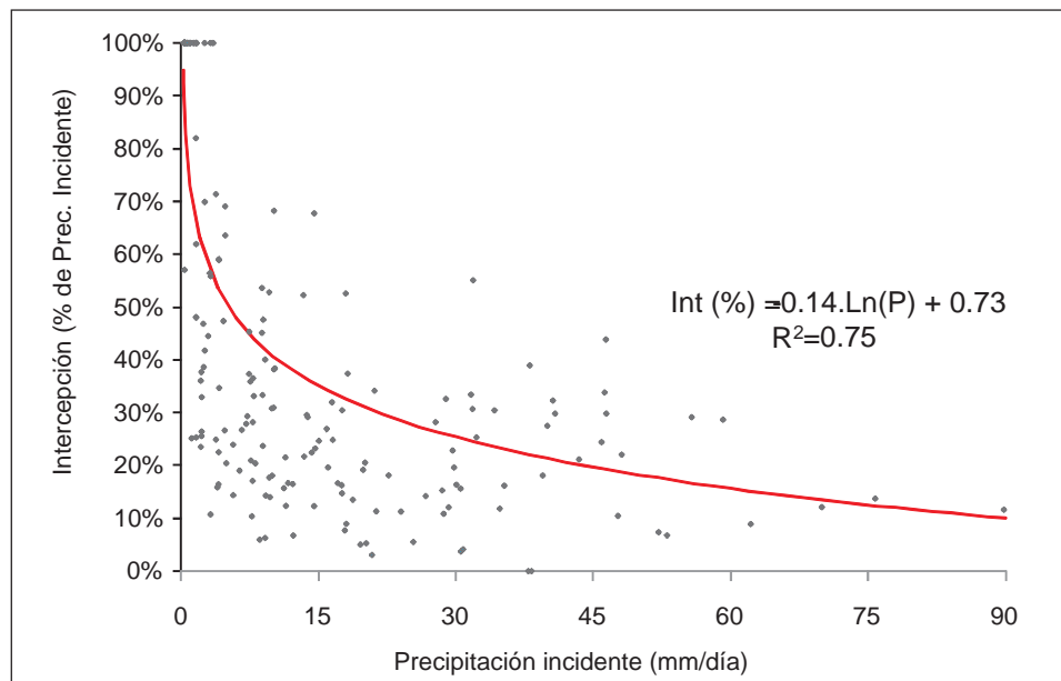
Figura 11. Relación entre la Intercepción y la precipitación total incidente para eventos diarios en la parcela Don Tomás.
