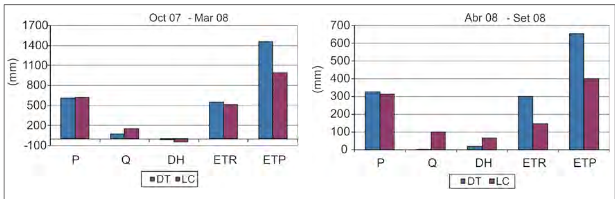
Figura 8. Balance hídrico estacional Oct 07 – Mar 08 y Abr 08 – Set 08.
