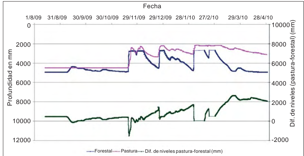
Figura 14. Recuperación de niveles piezométricos, ubicación media.
