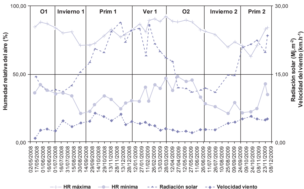
Figura 2. Dinámica temporal de los promedios de la humedad relativa del aire máxima (cruces) y mínima (círculos), radiación solar (triángulos) y velocidad del viento a 2 m de altura (rombos) entre fechas de muestreo. Campo Experimental 'La María', INTA EEA Santiago del Estero, 2008-09.
