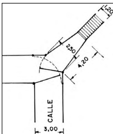
Medidas de un cargador tradicional.
