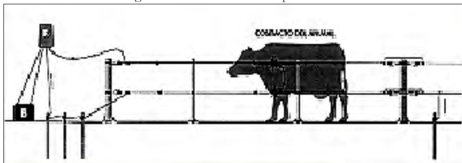
Figura 4. Retorno de tierra por alambre
