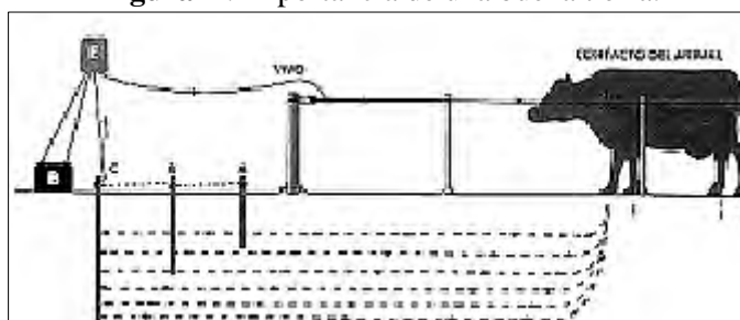
Figura 2 . Importancia de una buena tierra.
