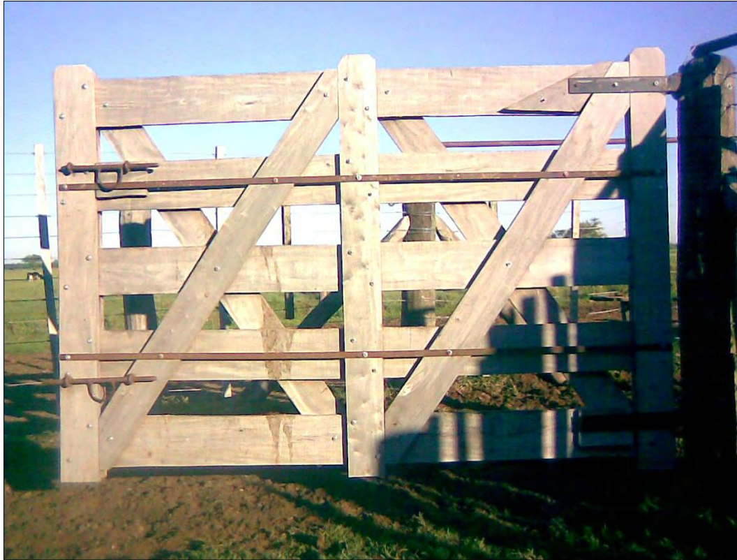
Portón común de tablas reforzado y con dos pasadores.
