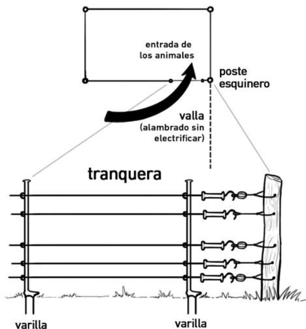
Figura 5. Vista superior de la parcela, donde se aprecia la ubicación de la tranquera y de la valla para facilitar la entrada de los animales al lote. Debajo se presenta una vista ampliada y detallada de la construcción de la tranquera.
