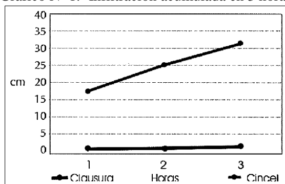
Gráfico N° 1.- Infiltración acumulada en 3 horas.
