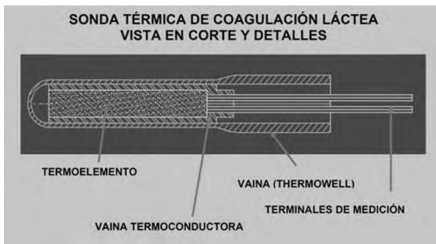
Figura 1. Corte esquemático del sensor.
