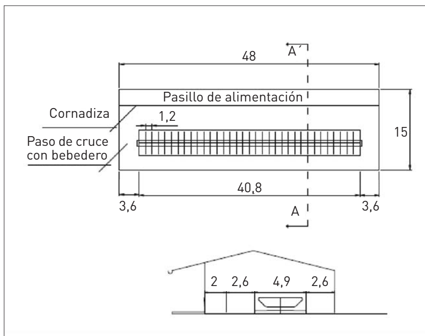
Figura 5: Croquis de una explotación en estabulación libre con cubículos.
