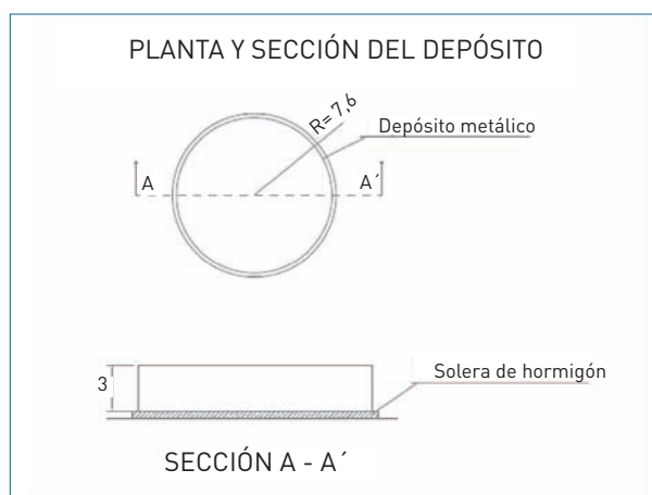
Figura 2: Fosa de purines circular.
