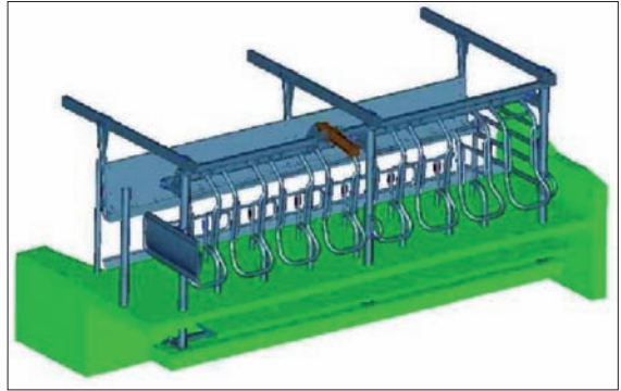
Figura 3. Sala tipo paralelo: esquema de barra delantera móvil y apertura automática.
