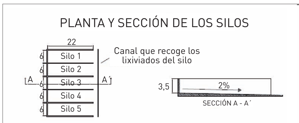
Figura 5: Silos trinchera.
