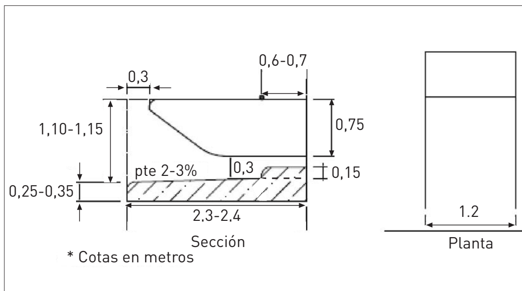
Figura 4: Medidas de un cubículo para vacas Holstein adultas.
