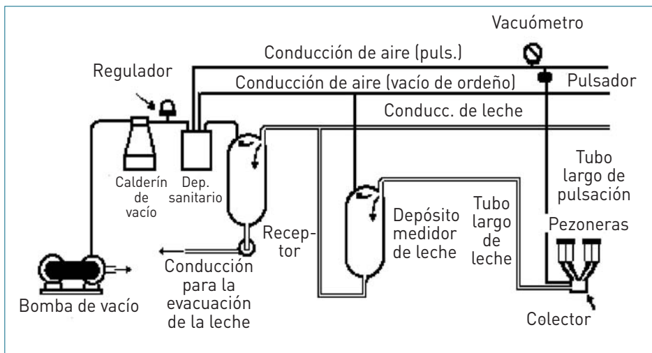
Figura 1: Componentes de máquina de ordeño con depósito medidor de leche.
