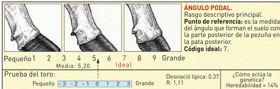
Figura 6: Ángulo podal.
