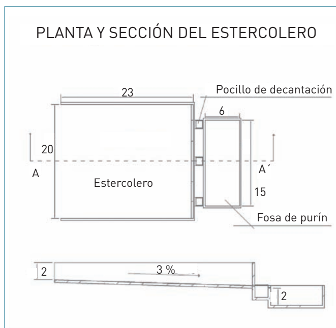
Figura 1: Estercolero con fosa de purín.
