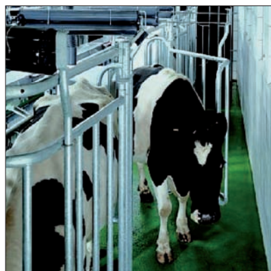
Figura 1: Sala tandem 4x2; distribución de boxes, foso y pasillo de salida.
