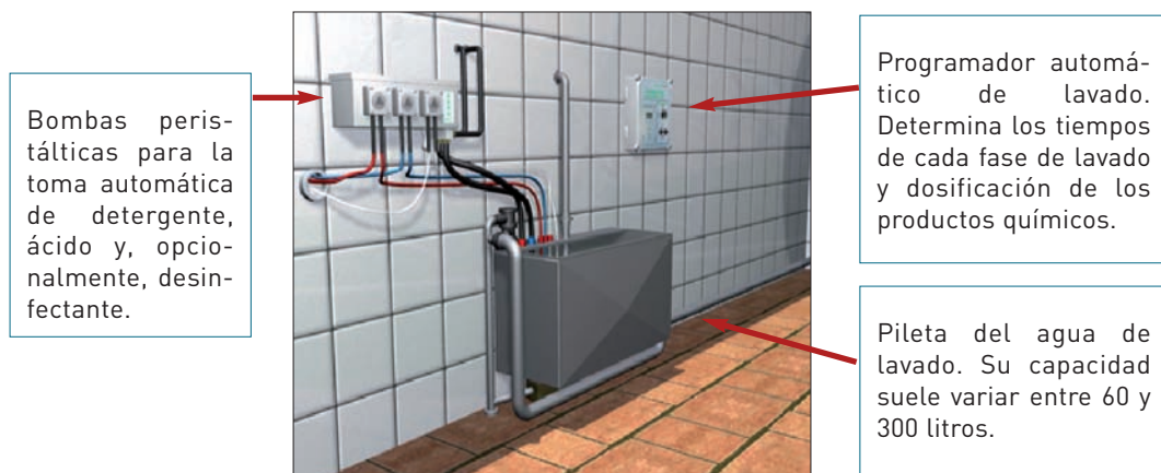
Figura 10: Imagen de un centro de lavado con sus componentes principales.
