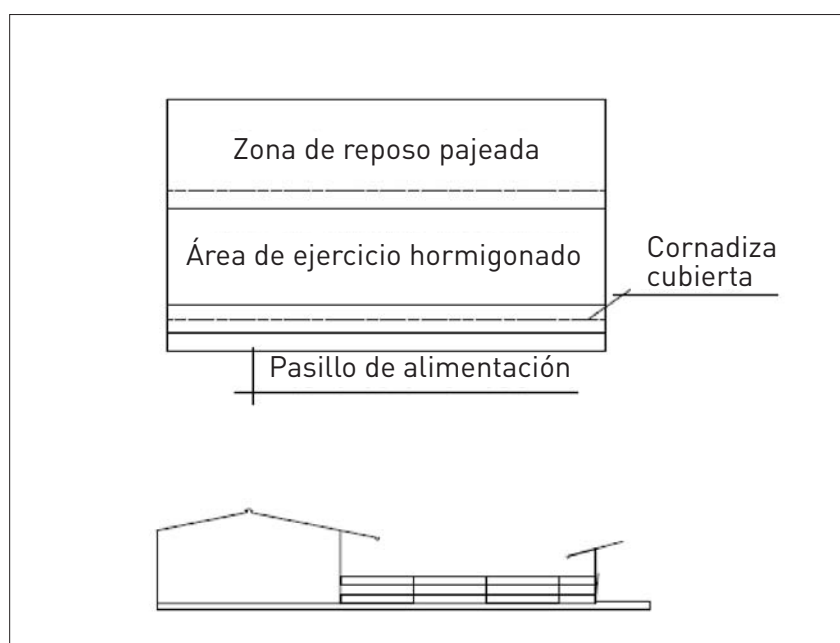
Figura 2: Planta y alzado de una estabulación libre.
