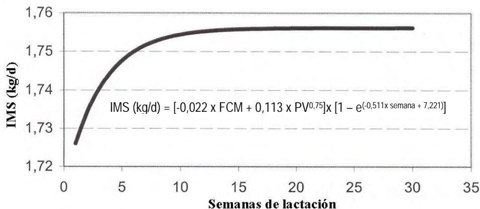
Figura 2.- Evolución del consumo de materia seca predicho por el modelo del NRC (2001) adaptado para cabras lecheras (2 kg FCM; 40 kg PV) (Fernández et al., 2003).
