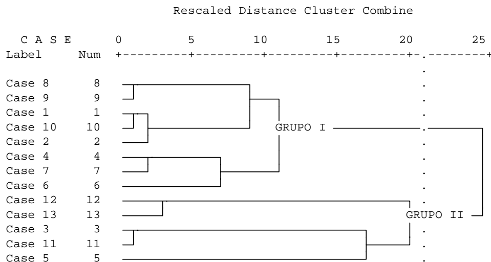
Figura 2. Dendrograma usando método de Ward. (Dendrogram using Ward method).
