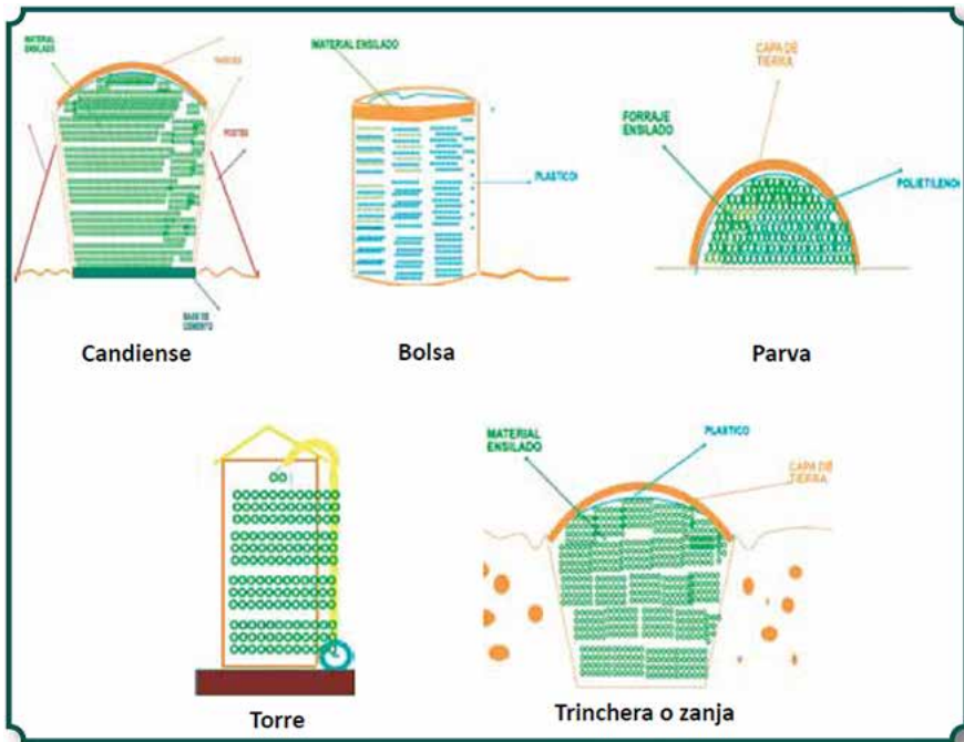
Figura 3.1. Diferentes tipos de silo.
