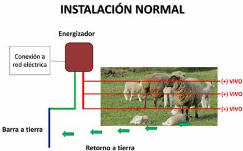
Figura 8.5. Generador y cable a tierra de un sistema de cerco eléctrico.
