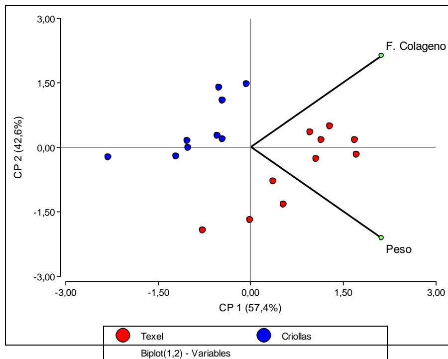
Gráfico 1. Biplot de las variables y los ovinos discriminados según raza.
