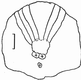
Fig. 5. — Escama latinucleada del flanco dorsal, con radios, y tres regeneraciones parciales.
