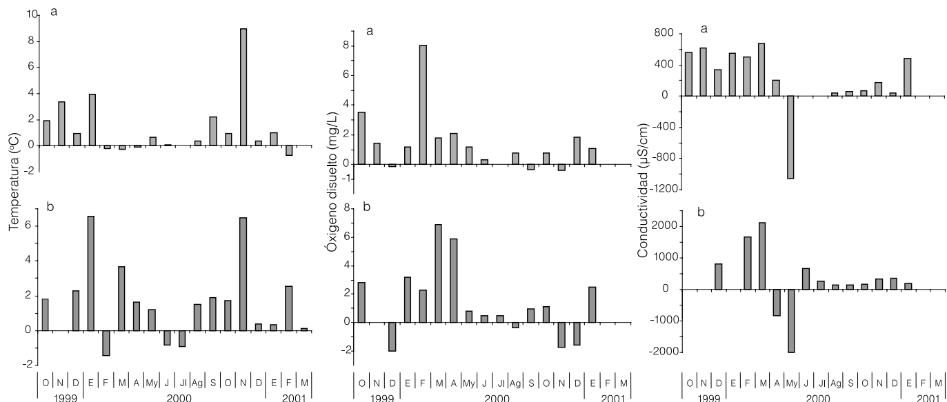
Figura 6. Dinámica temporal de la diferencia en la temperatura ( ^{\circ}\text{C} ), el oxígeno disuelto ( \text{mg/L} ) y la conductividad eléctrica ( \mu\text{S/cm} ) del agua entre el ambiente litoral y el pelágico en ambos sitios de estudio. a: costa vegetada, b: costa de tosca.
