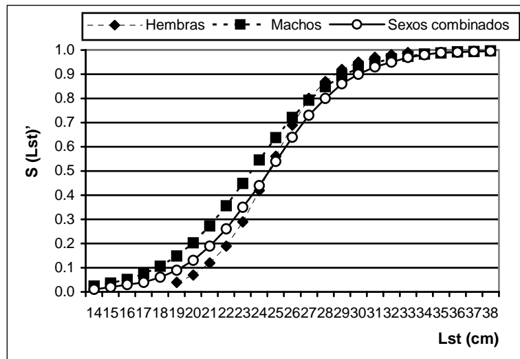
Figura 13. Frecuencias relativas acumuladas suavizadas S(Lst)' de ejemplares de trucha arco iris adultos machos, hembras y sexos combinados por intervalos de talla para el RDLP.
