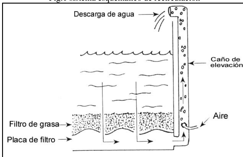
Fig.1 sistema esquemático de recirculación
