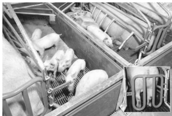
Figura 15: Jaula paridera. Detalle de la barra de protección en forma de peine.
