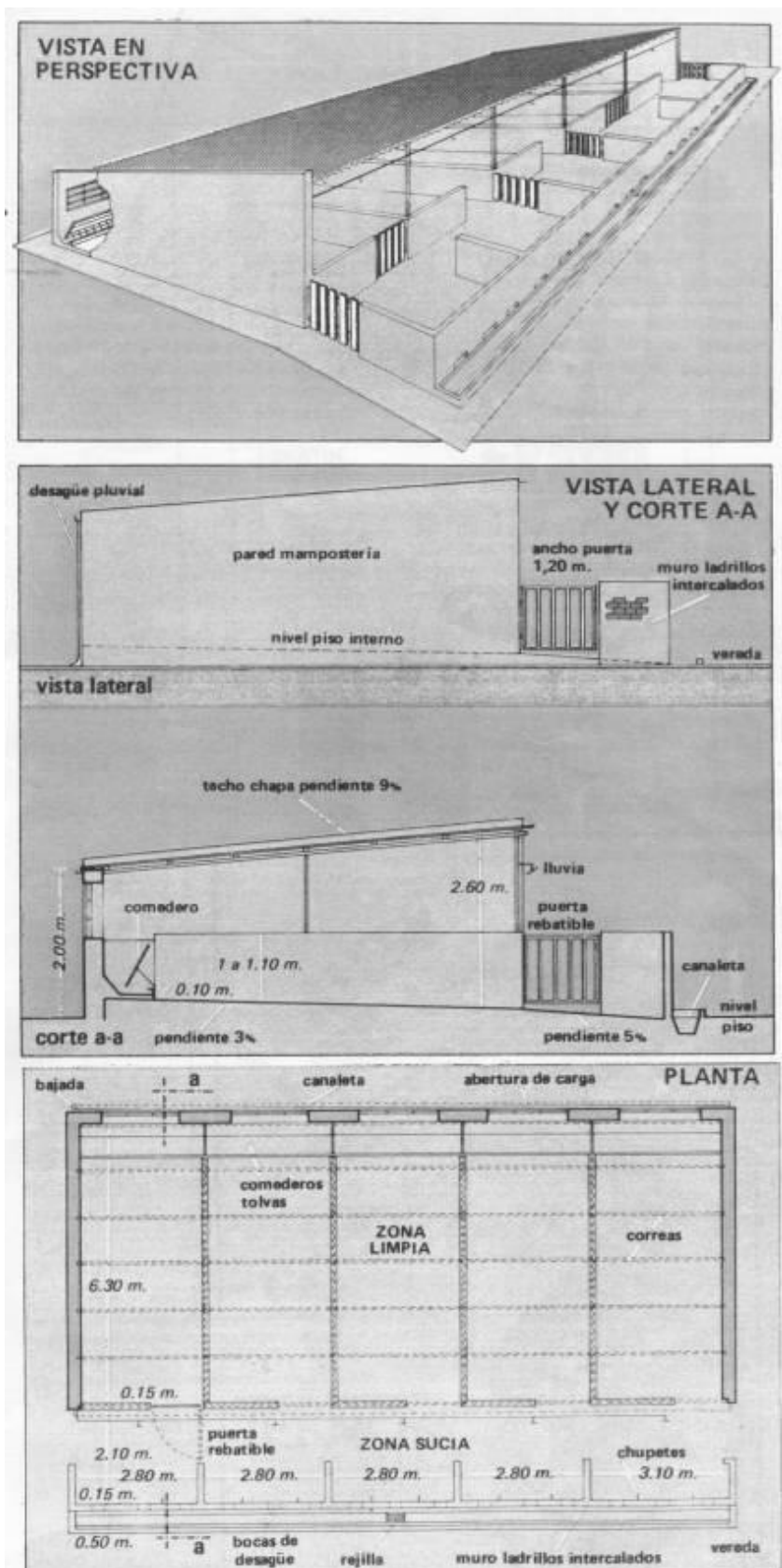
Figura 26: Pista de frente abierto. Detalle constructivo.
