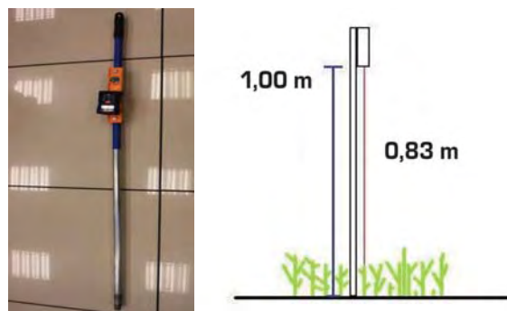
Figura 2. Telémetro láser y su funcionamiento.
