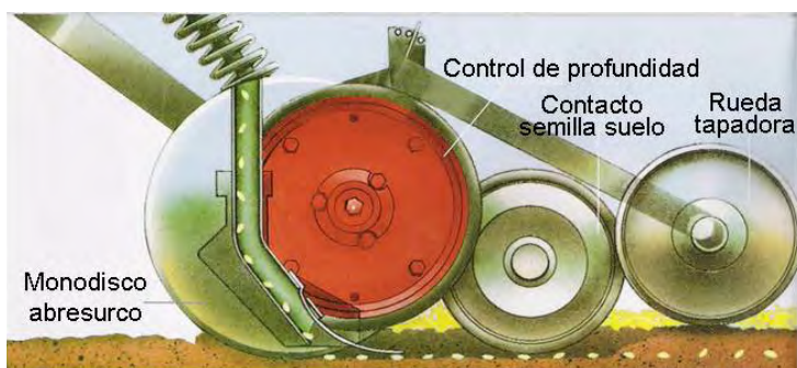
Figura 1. Abresurco monodisco.
