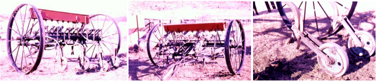
Maquina casera para intersementar, muy sencilla (Establ. Oscar Najles, Alpa Corral, Córdoba).
