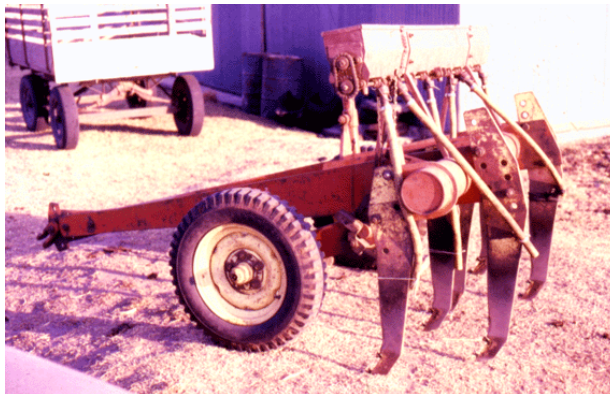
Intersementadora fabricada con un subsolador (Los Cerros, de Rita, La Barranquita)
