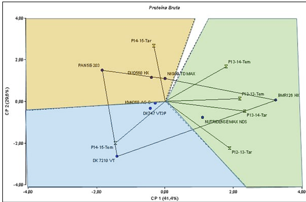
Gráfico 4: Biplot GG para el contenido de Proteína Bruta de los ocho cultivares de maíz evaluados en los seis ambientes.
