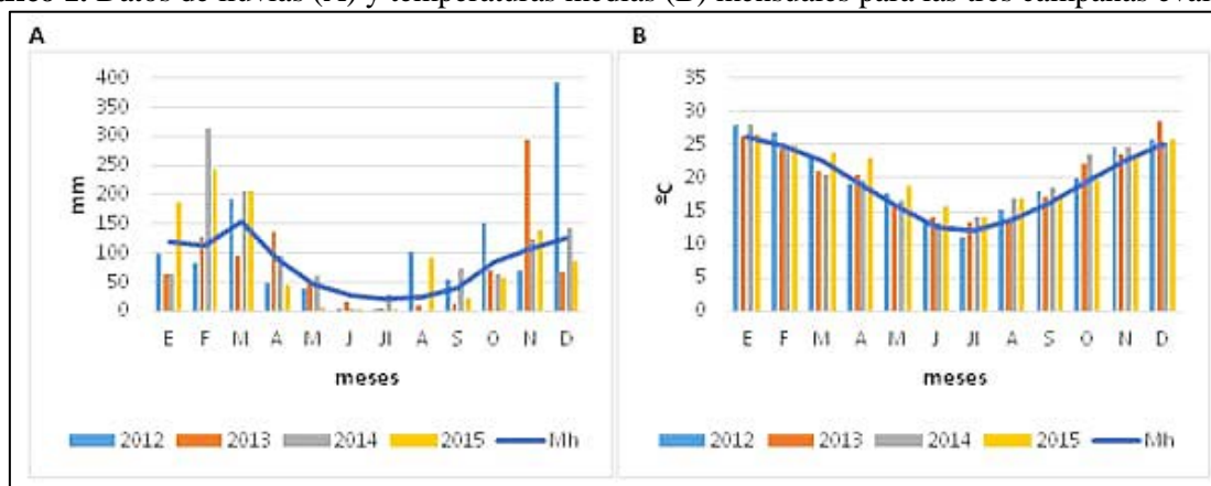
Grafico 1. Datos de lluvias (A) y temperaturas medias (B) mensuales para las tres campañas evaluadas
