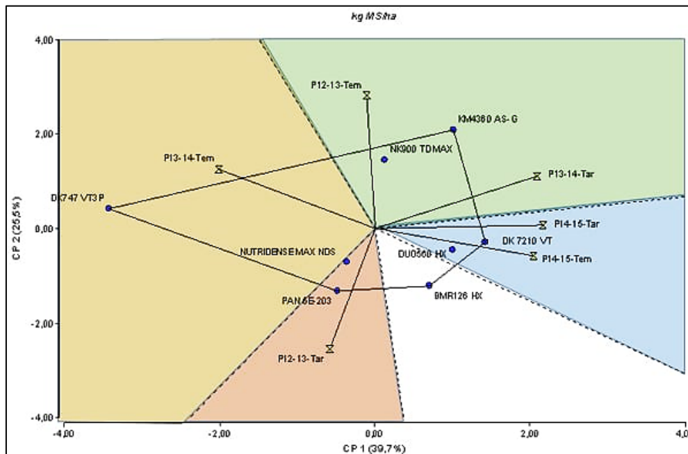
Gráfico 1: Biplot GG para el rendimiento en Materia Seca de los ocho cultivares de maíz evaluados en los seis ambientes.
