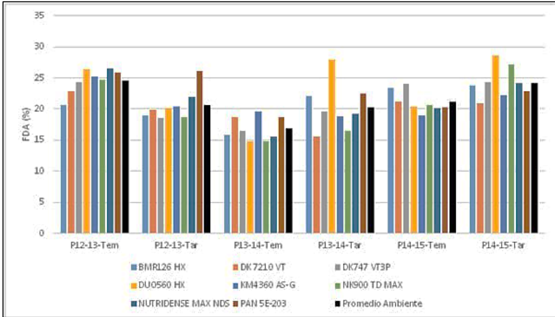
Grafico 6: Contenido promedio de FDA (%) de los ocho cultivares de maíz evaluados en las tres campañas, dos épocas de siembra y el promedio general para el ambiente.
