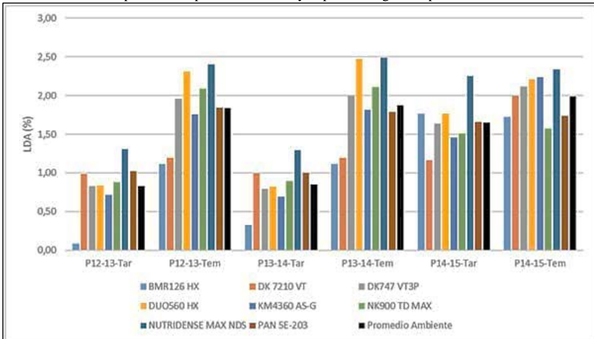
Grafico 7: Contenido promedio de LDA (%) de los ocho cultivares de maíz evaluados en las tres campañas, dos épocas de siembra y el promedio general para el ambiente.
