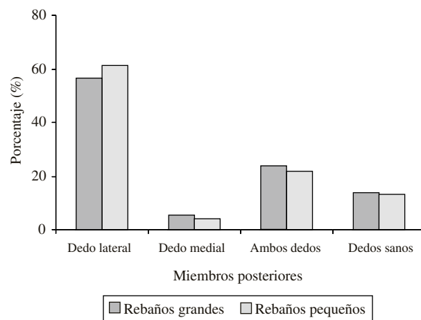
Figura 4. Distribución de las lesiones (%), de acuerdo al dedo afectado en los miembros posteriores de las vacas examinadas, en 34 rebaños grandes (n = 676) y 57 pequeños (n = 422) de la Décima Región, Chile.
