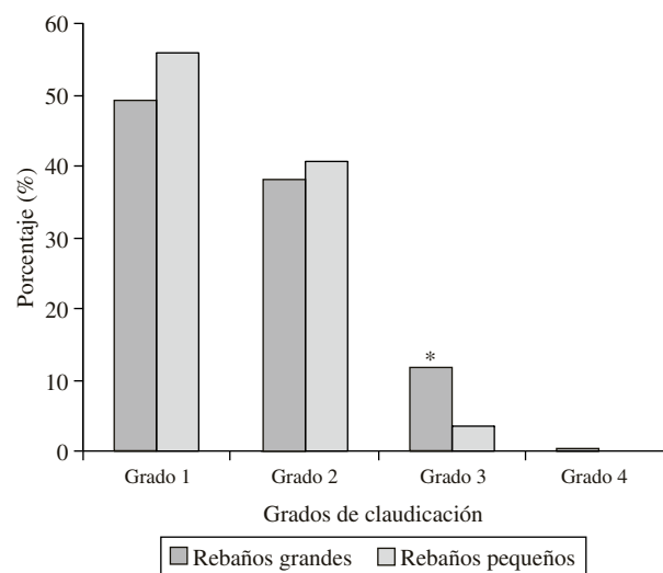
Figura 2. Distribución de los grados de claudicación (%) en vacas cojas de 34 rebaños grandes ( n = 3.014 ) y 57 rebaños pequeños ( n = 458 ) de la Décima Región, Chile. * P < 0,037 .
