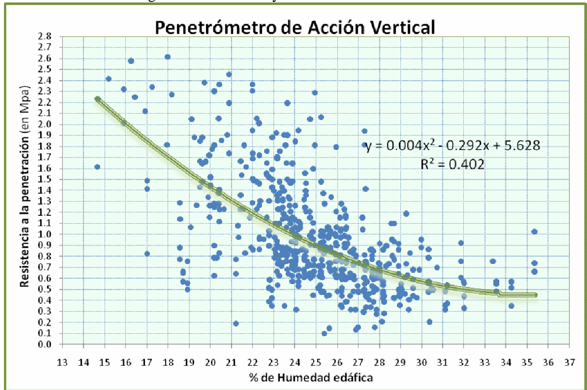
Gráfico 1. Curva de regresión entre la RP y la humedad.
