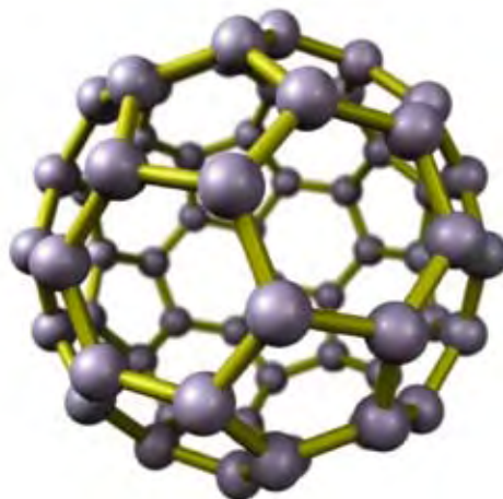
Figura 2. Fullereno.
