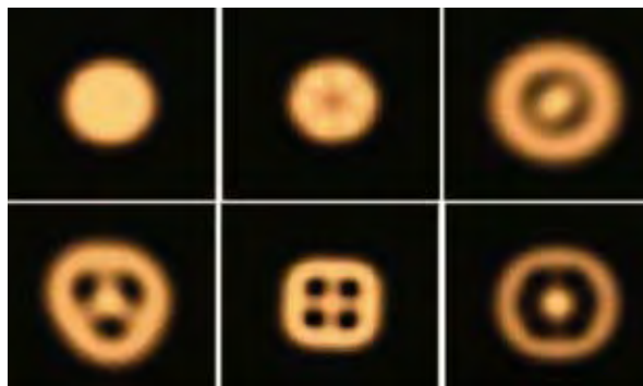
Figura 5. Puntos cuánticos.
