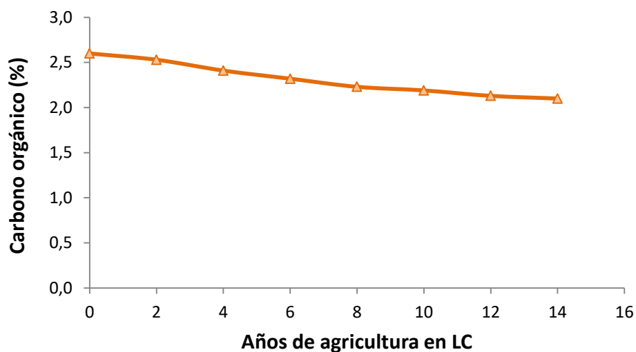
Figura 1- Variación del contenido de Carbono orgánico en la capa arable de un suelo Argiudol petrocalcico en la zona de Tres Arroyos con labranzas. a) bajo pastura y b) bajo agricultura luego de una pastura.
