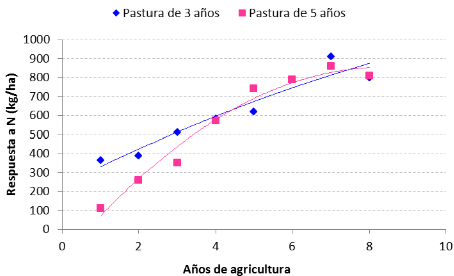
Figura 3: Respuesta a fertilización nitrogenada en trigo luego de un período de 3 y 5 años de pastura. Fuente: Ensayos de rotaciones con labranzas CEI Barrow
