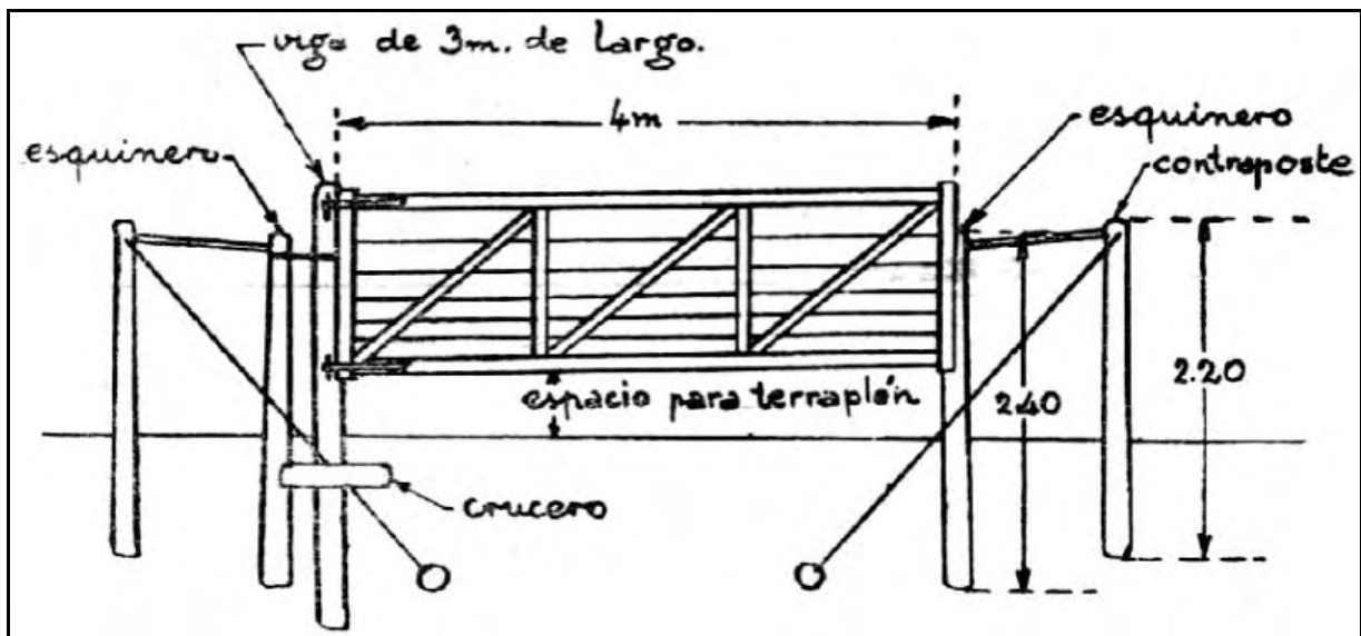
Colocación de una tranquera de madera.
