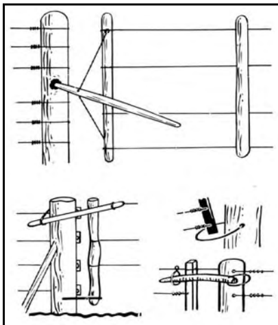
a)-Distintos tipos de cierre para tranqueras de alambre. b)-Un tipo de cierre para tranquera de madera.
