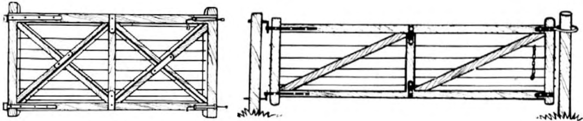
Tranqueras de madera de tirantes y hierro redondo; a) reforzada para corrales; b) común para potreros.
