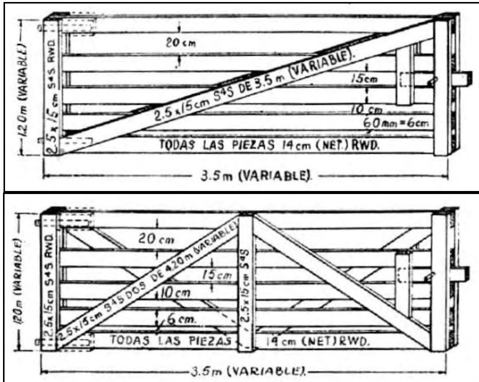
Tranqueras de tablon.
