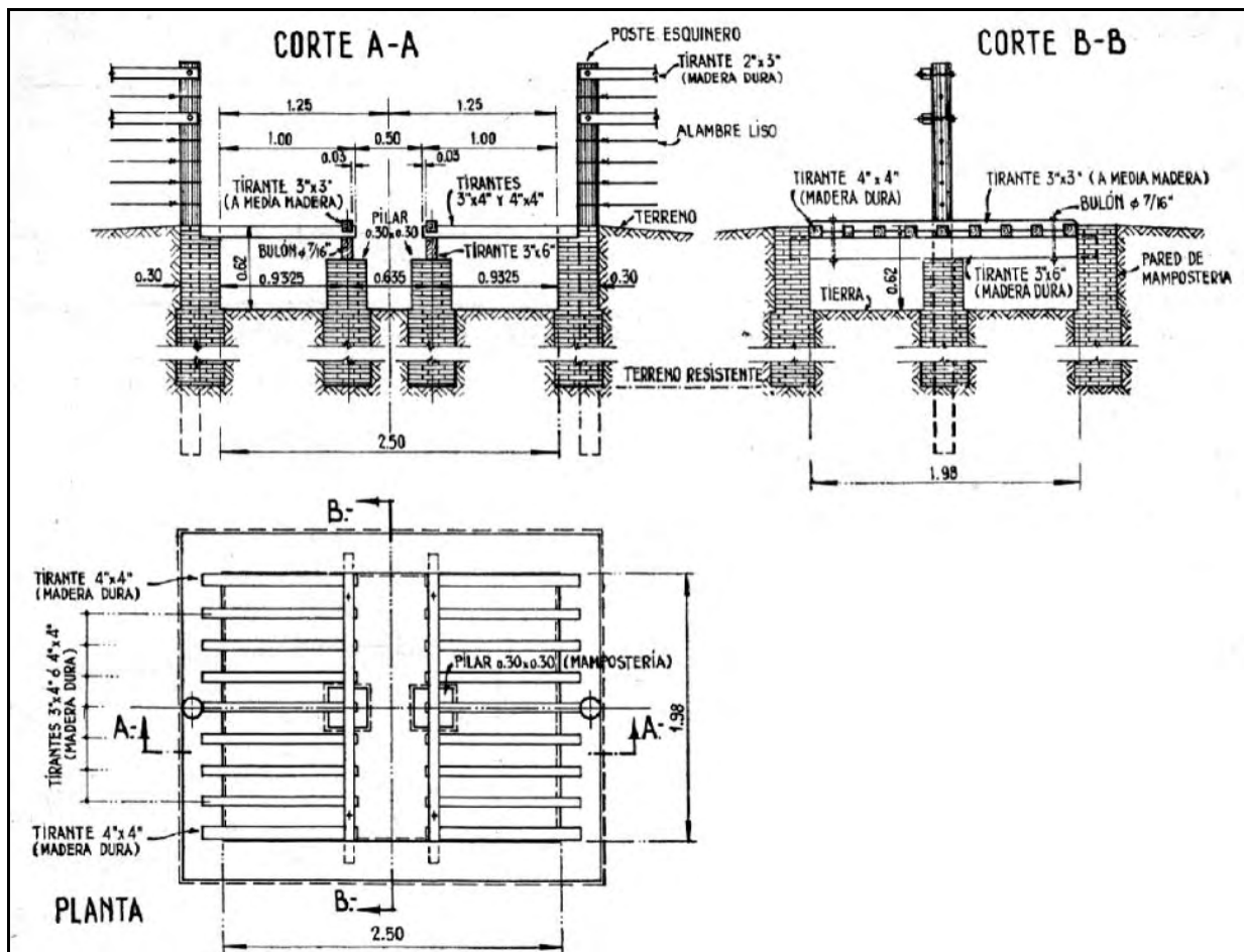
Croquis de guardaganado (sin escala)
