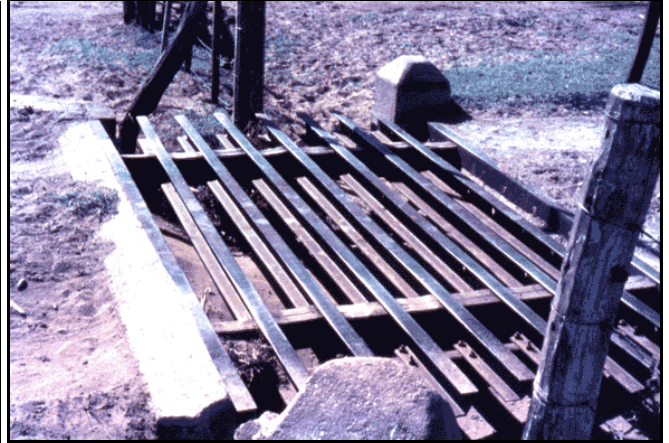
a)-Guardaganado con tranquera automático. Cuando el vehículo presiona el piso, la tranquera se eleva inmediatamente.
