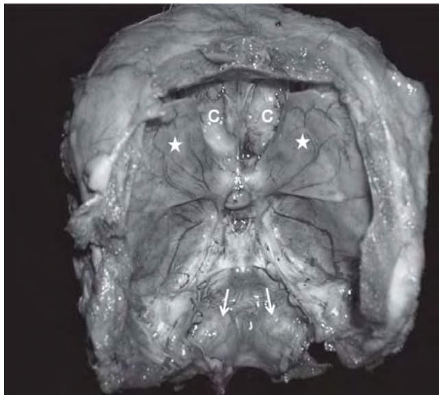
Figura 4. Deformaciones óseas severas en interior de la cavidad craneana (Caso 2). Se destacan las imperfecciones de lamina cribosa (C), alas del presfenoides salientes (estrellas) y constricción de la pars basilaris por engrosamientos internos de cóndilos occipitales (flechas).
