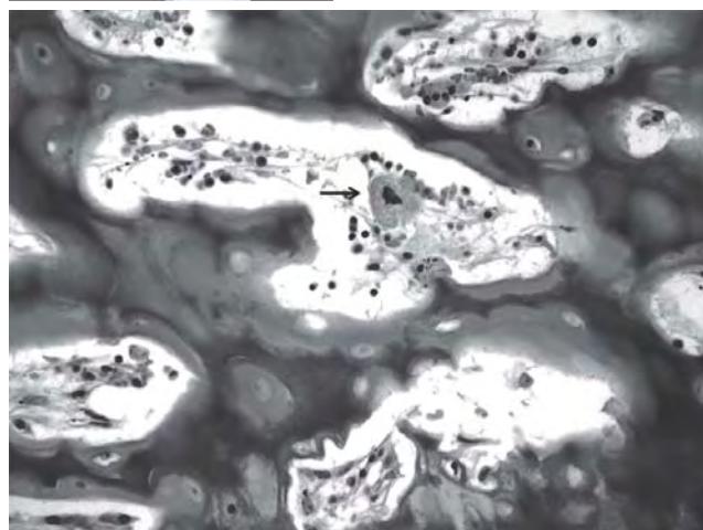
Figura 7. Corte histológico de metáfisis distal de húmero (Caso 1). Se observan las trabéculas condro-óseas interconectadas, los osteoclastos necróticos (flecha) y la ausencia de lagunas de Howship. H&E, 400x.
