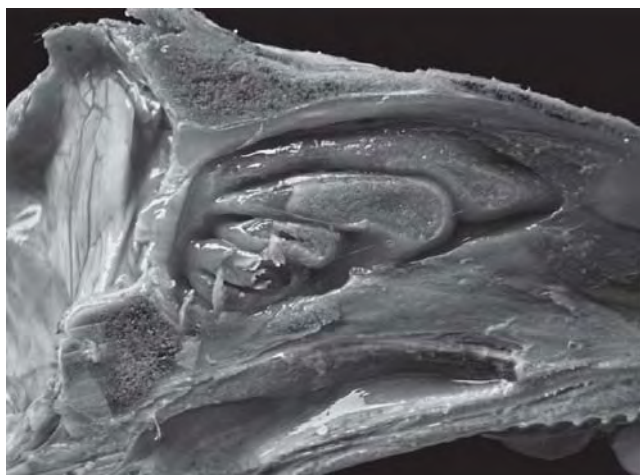
Figura 5. Corte sagital de cráneo mostrando ausencia de senos esfenopalatino y senos frontales y cornetes nasales grandes obstruyendo los pasajes aéreos (Caso 2).
