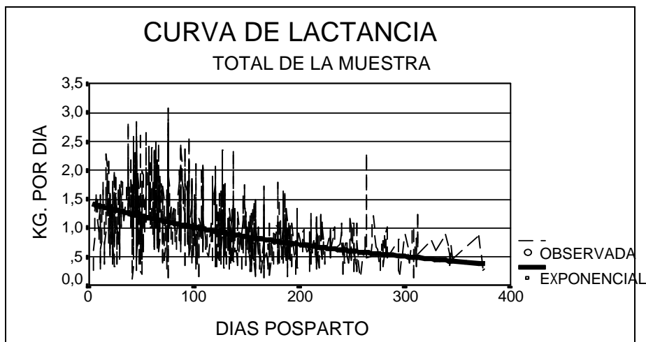
Gráfico V-15: Dispersión Simple entre producción de leche (kg. por día) y días posparto con ajuste de curva.
