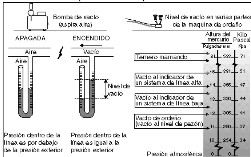
Figura 2: El nivel de vacío es medido conforme la altura de la columna de mercurio (0 kilo Pascales) cuando el aire es aspirado fuera del espacio en donde se mantiene.
