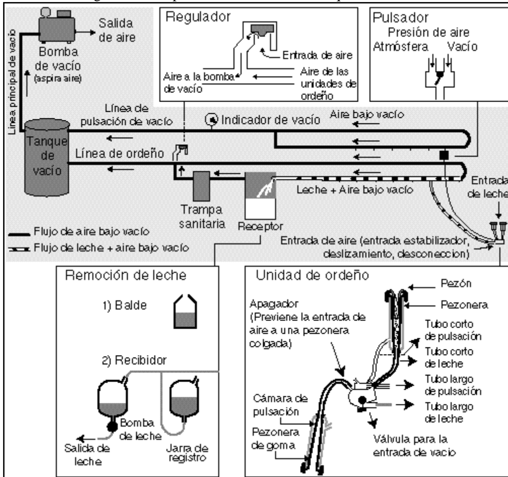
Figura 1.- Componentes básicos de las máquinas de ordeño
