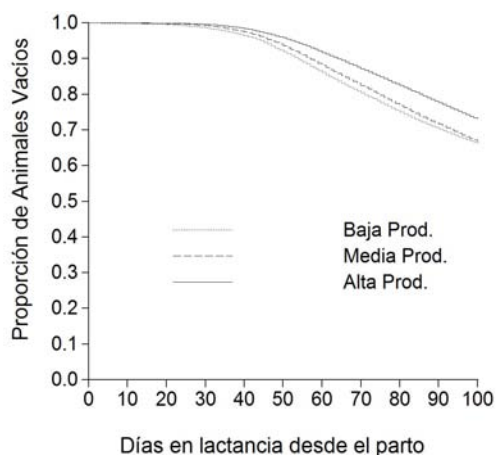
Figura 7. Curva de sobrevivencia de Kaplan-Meier. Días en lactancia que transcurren hasta lograr la preñez para lactancias con distintos niveles productivos. Estadístico Chi-cuadrado para media vs. baja: 13.275 ( p=0,0002 ); estadístico chi-cuadrado para media vs. alta: 539,0 ( p<0,0001 ) y estadístico chi-cuadrado para baja vs. alta: 702,080 ( p<0,0001 ).
