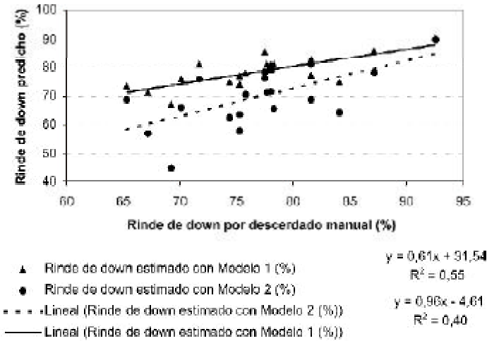
Figura 2: Relación entre rinde de down por descardado manual y rinde de down predicho por dos modelos. Modelo 1 sin corrección por largo de fibras y Modelo 2 con corrección por largo de fibras. La densidad de pelos en ambos casos es de 1,31 g/cm 3 .
